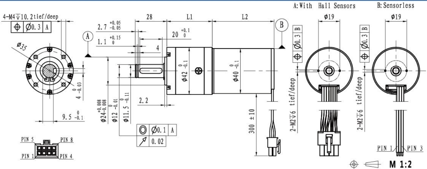
ECG40..L ECG40..S P42
